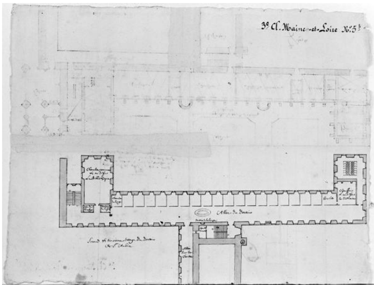
Dessin du dortoir à bâtir à Saint-Aubin, fait par Dom Journeaux... Second et troisième étage : plan aux 2 e et 3 e étages de l'aile est, projet, Lavis, 1674, éch. 1 : 243. (Archives nationales ; N III Maine-et-Loire 5/3, verso).
