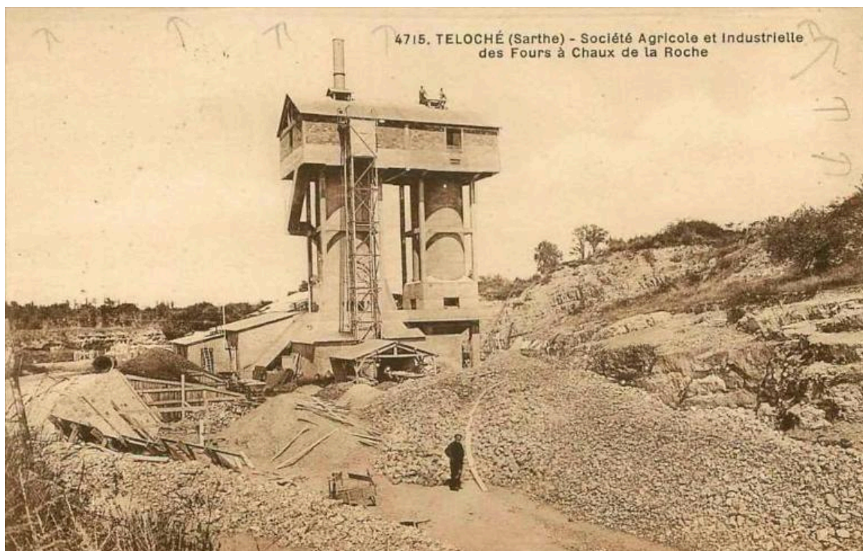
Four à chaux, 1930.
