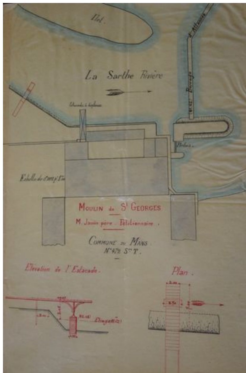
Plan général de la minoterie.
