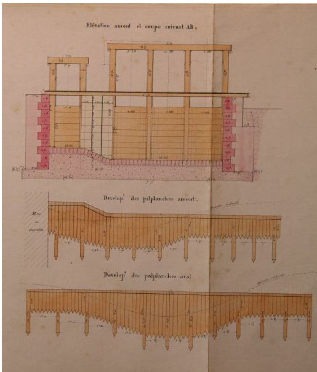
Élévation amont et coupe suivant AB.
