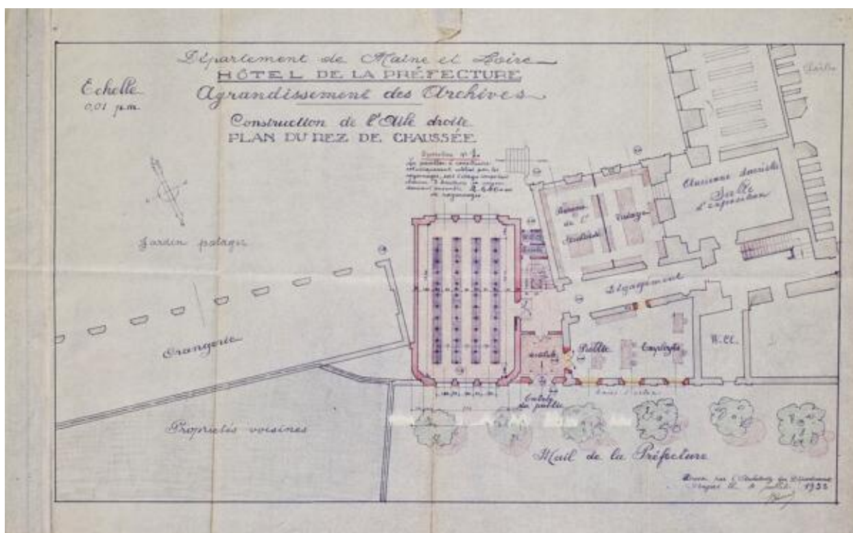
Département de Maine-et-Loire. Hôtel de la Préfecture. Agrandissement des Archives. Construction de l'aile droite. Plan du rez-de-chaussée, par Ernest Bricard, 30 juillet 1933, éch. 1:100e. (Archives départementales de Maine-et-Loire ; 48 alpha 34);
