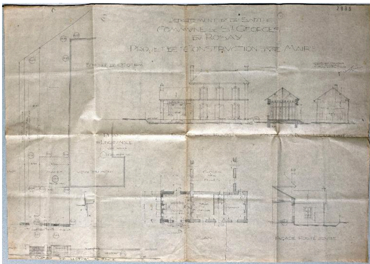
Plans, coupes et élévations de l'école et de la mairie projetée. 1926.
