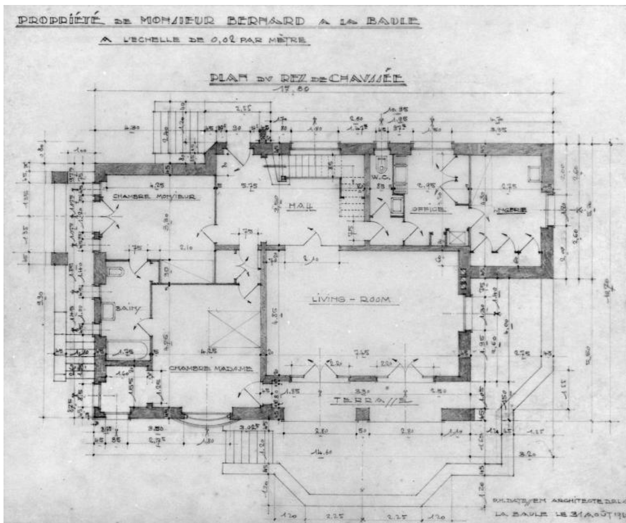
Plan du rez-de-chaussée au 1/50e de la villa Soladar pour M. Bernard.
