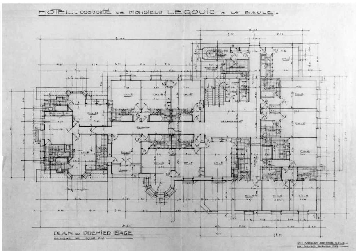
Plan du 1er étage au 1/50e du Celtic Hôtel pour Monsieur Le Gouic en 1929.
