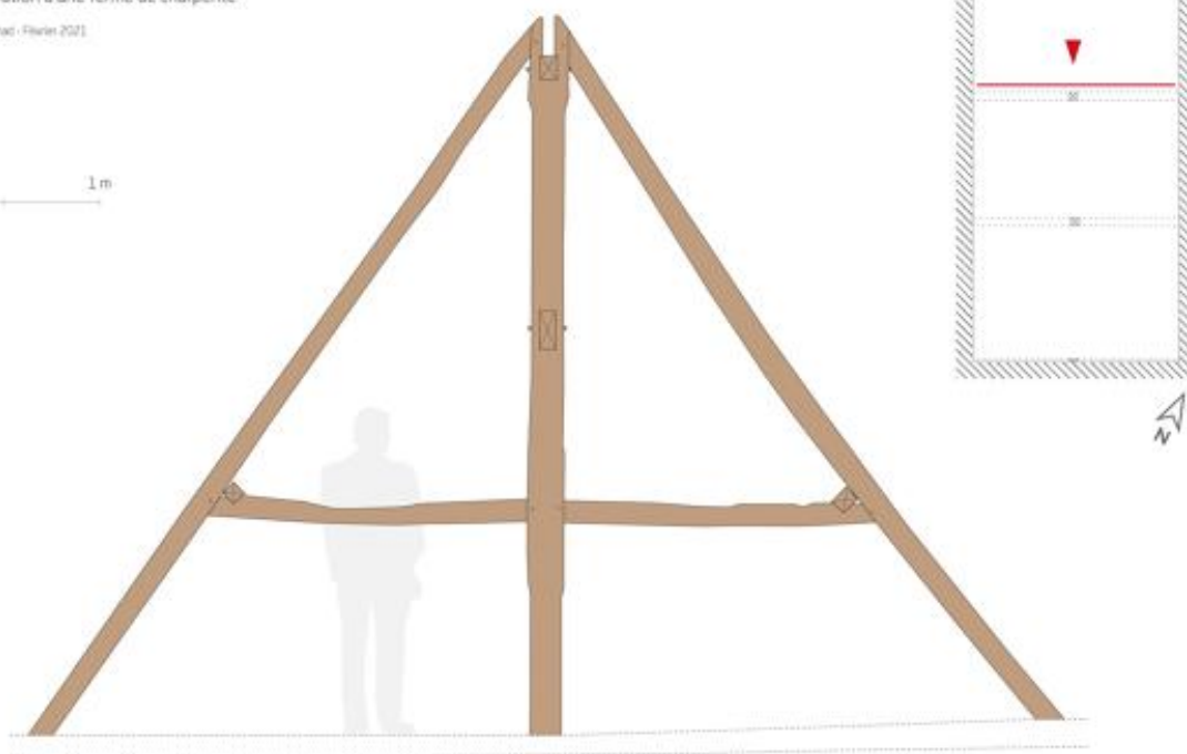
LE MANS (72) - Saint-Georges-du-Plain - Ancien presbytère de l'église Saint-Georges Relevé d'élévation d'une ferme de charpente
