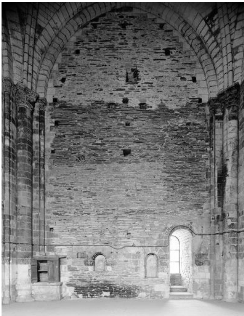
Tour-clocher dite tour Saint-Aubin, salle haute : élévation intérieure ouest. A gauche, le puits.
