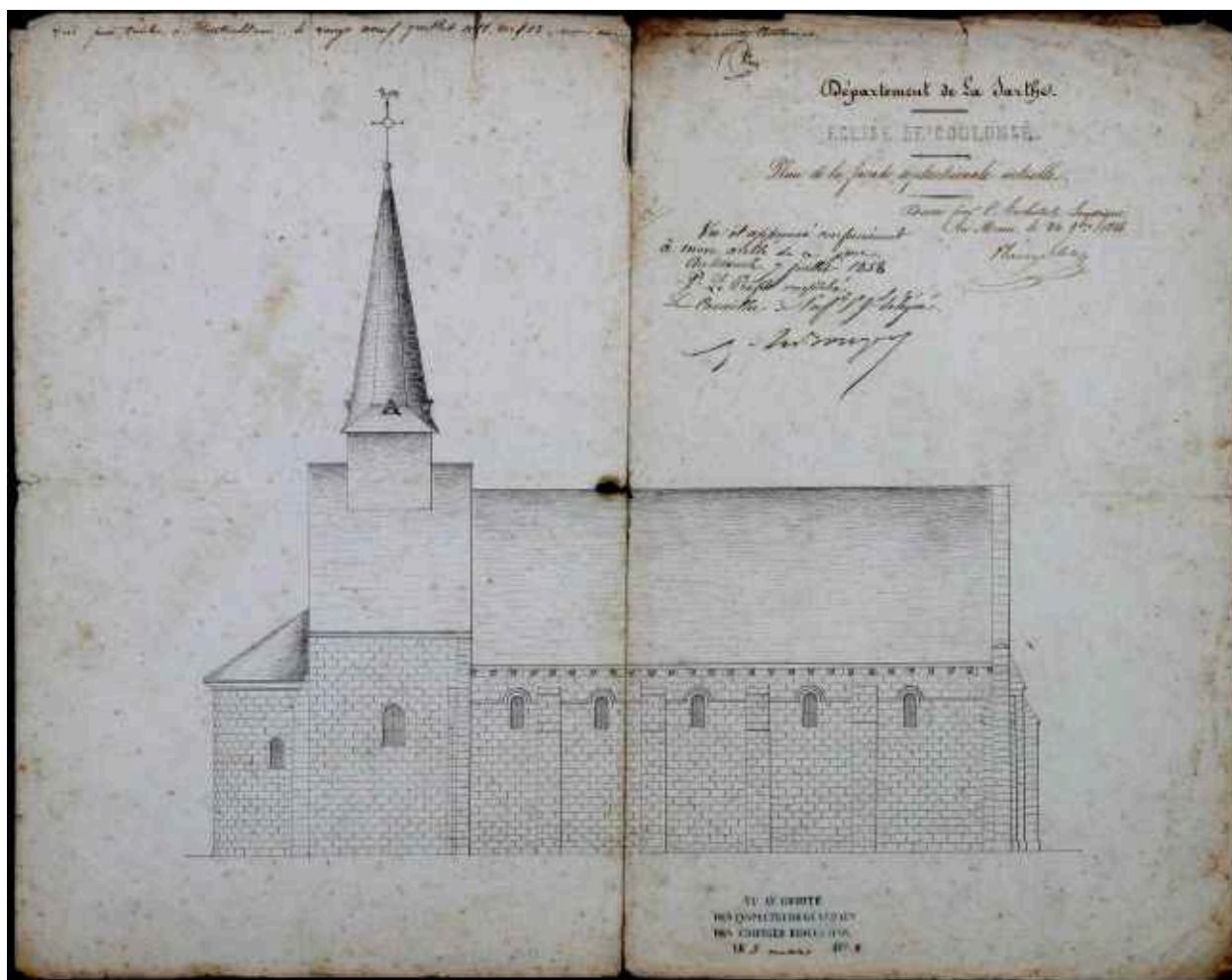
Élévation de la façade septentrionale avant restauration, 1858.
