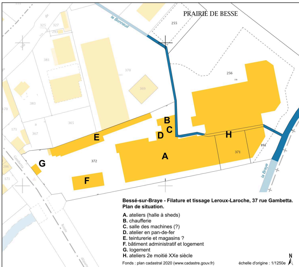
Plan de situation de l'usine textile Leroux-Laroche à Bessé-sur-Braye.
