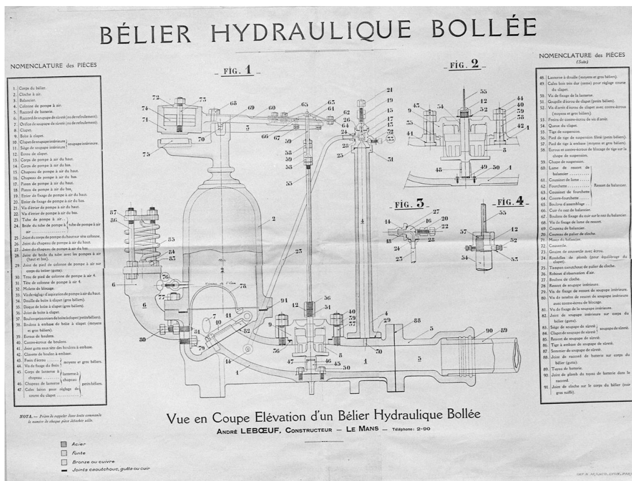
Vue en coupe. Elévation d'un Bélier Hydraulique Bollée, 1ère moitié du XXe siècle.
