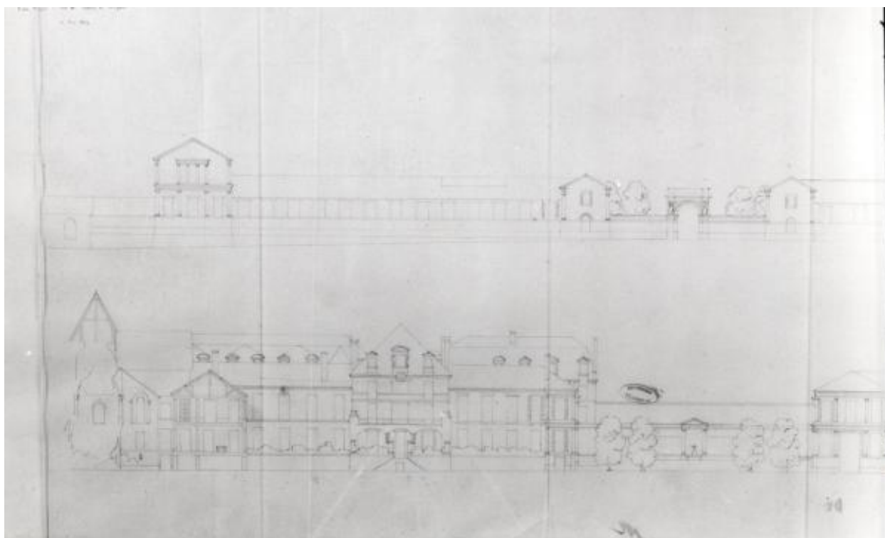
Maine-et-Loire. Ecole royale d'arts et métiers à Angers, vu mai 1842 : élévation des bâtiments sur la rue du Godet et à hauteur du logis abbatial. Détail sur la partie gauche du document, comprenant le logis abbatial.
