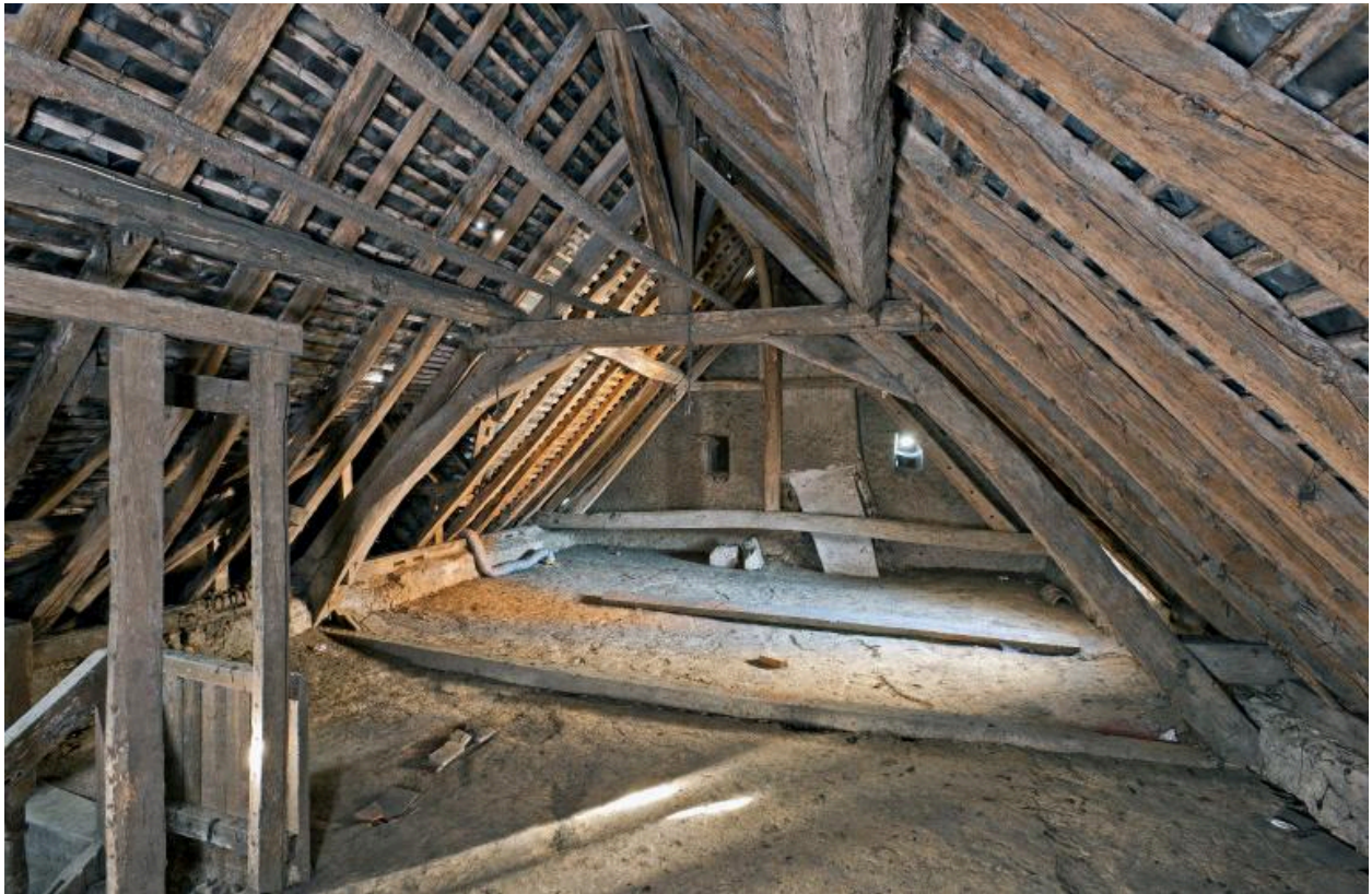
Charpente du comble de la maison sur rue.
