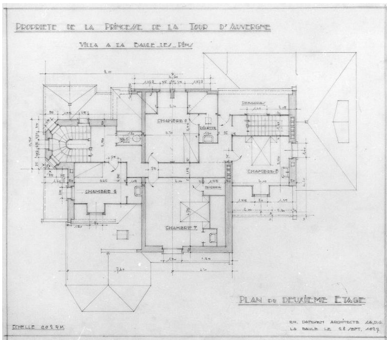
Plan du 2e étage au 1/50e du projet de villa pour la princesse de La Tour d'Auvergne en 1927
