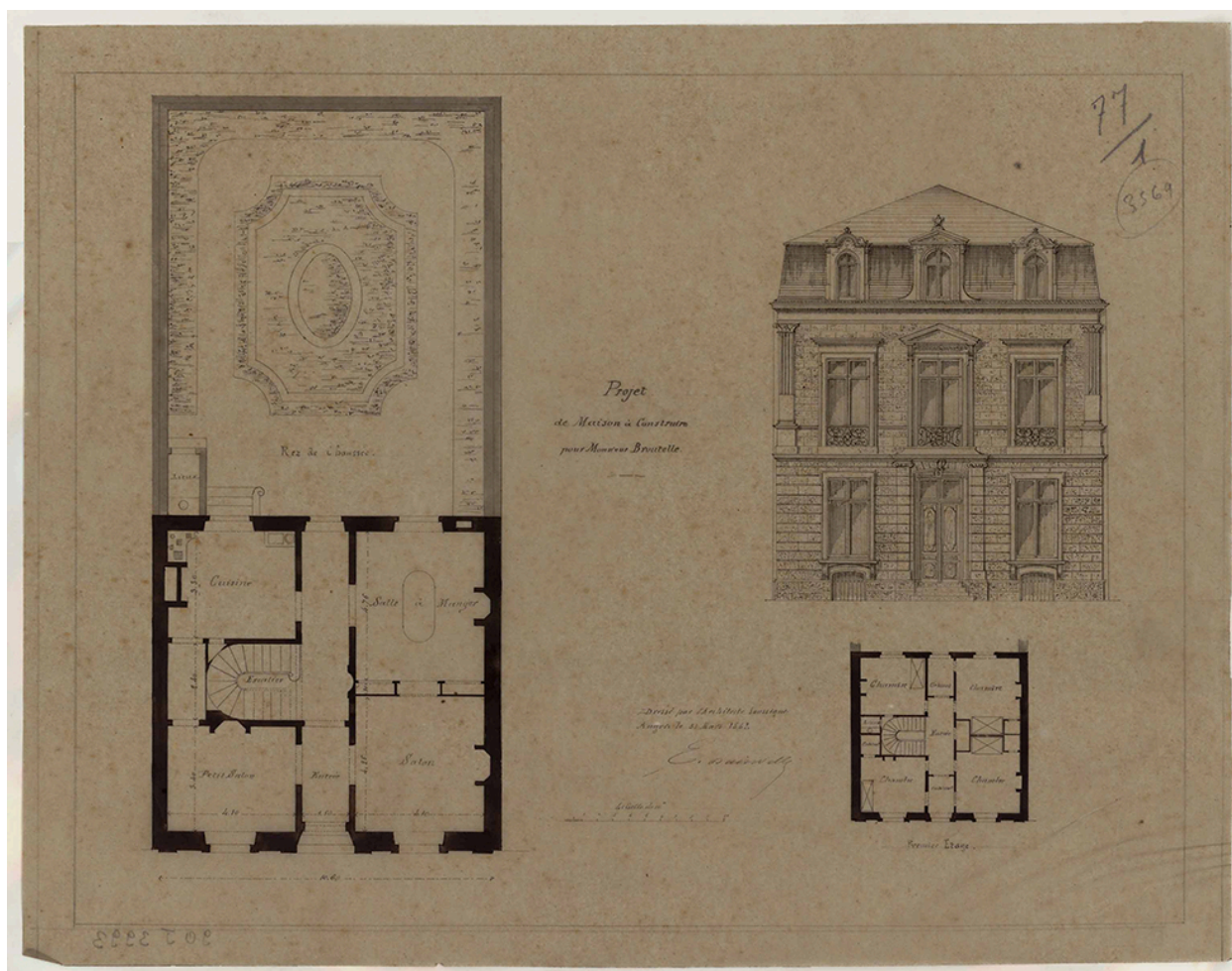
Maison d'habitation appartenant à Monsieur Broutelle. Élévation de façade principale, plan du rez-de-chaussée et du 1er étage. 1862. (AD Maine-et-Loire ; 90 J 3993).
