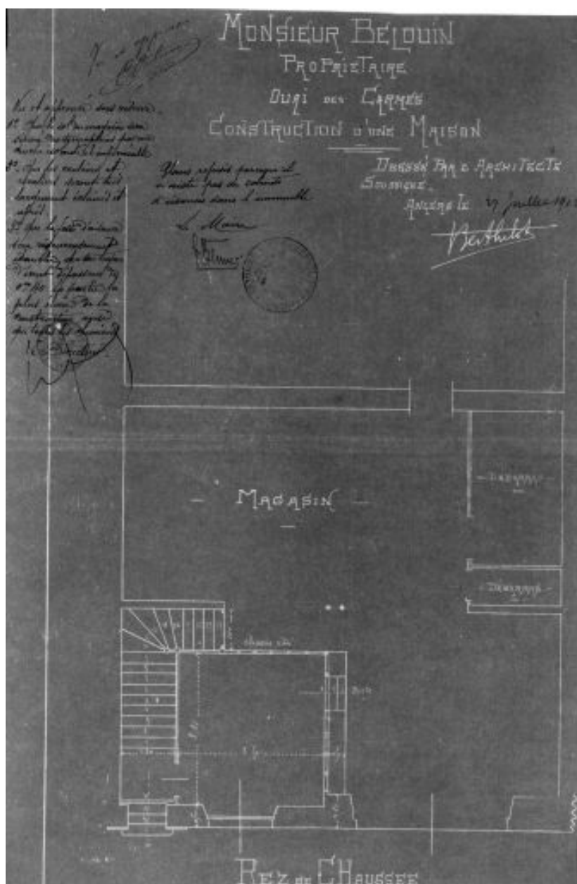
Plan du rez-de-chaussée, relevé pour le permis de construire, par J.-A. Berthe, 1912.
