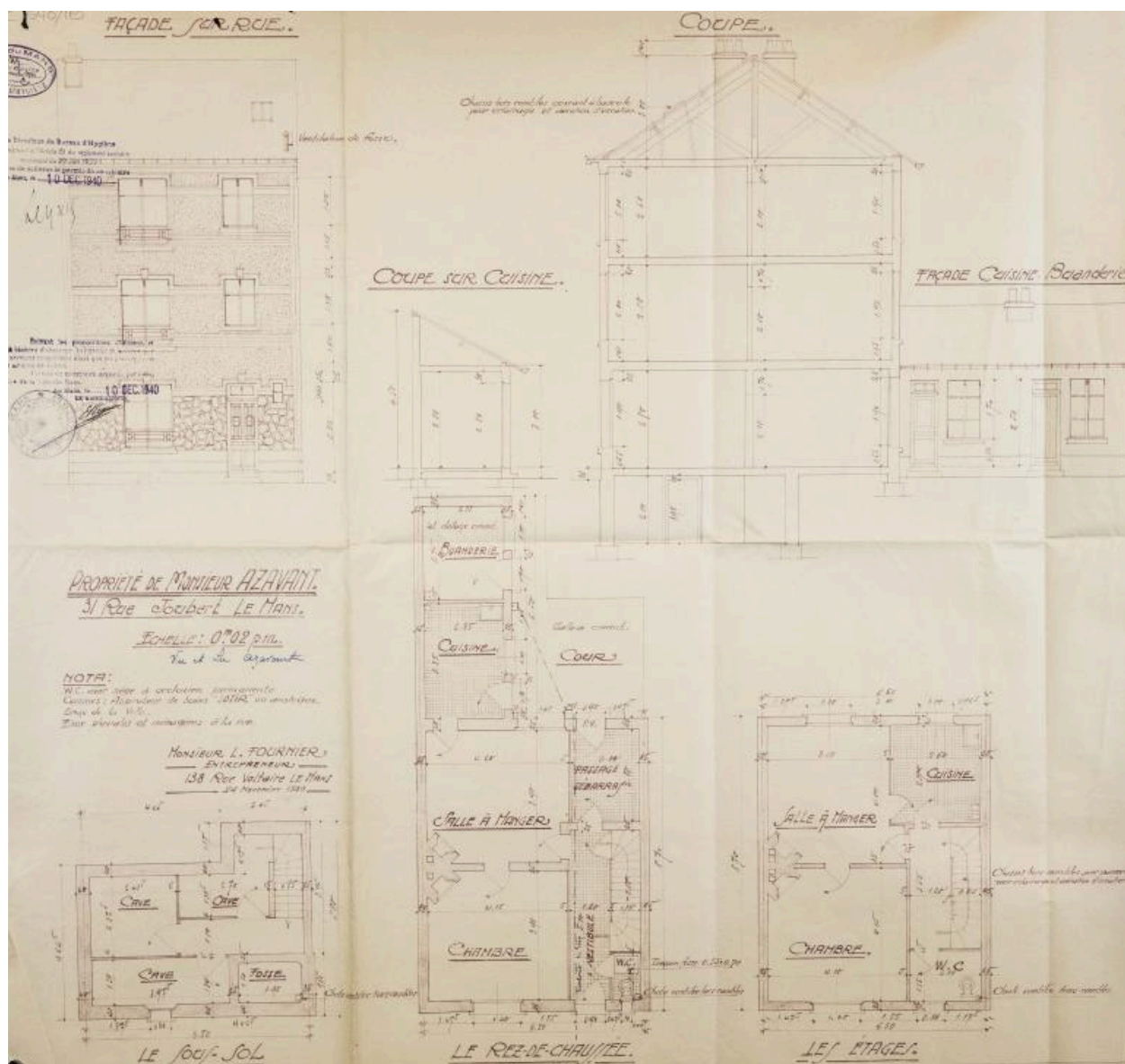
Plan, coupe et élévation d'une maison rue Joubert.
