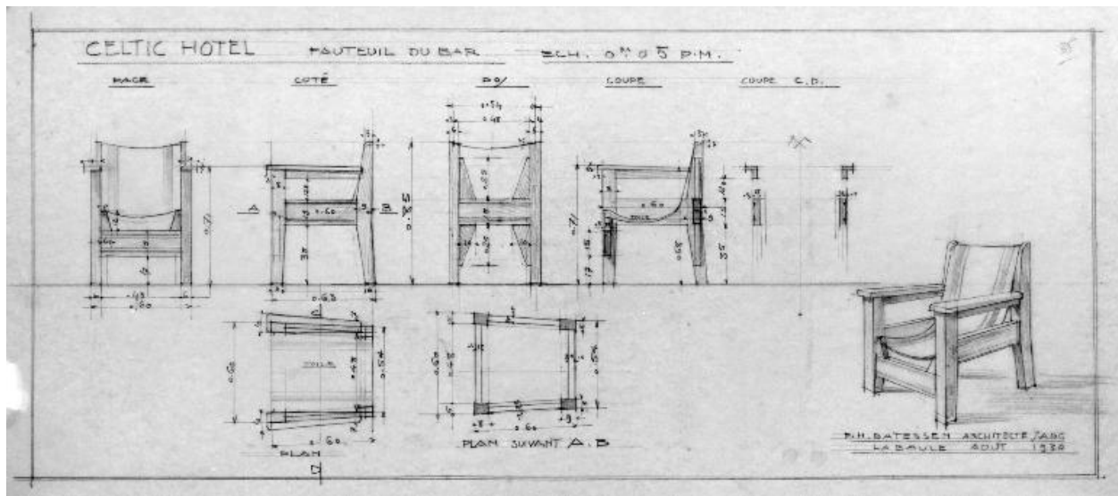
Dessins au 1/20e des fauteils du bar du Celtic Hôtel pour Monsieur Le Gouic en 1930.
