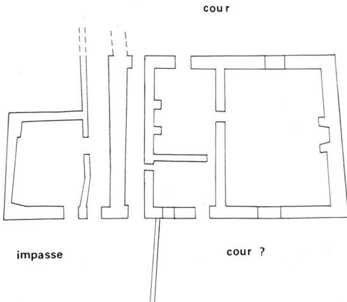
Plan du rez-de-chaussée d'après le plan Dainville de 1877, éch. 1 : 125.
