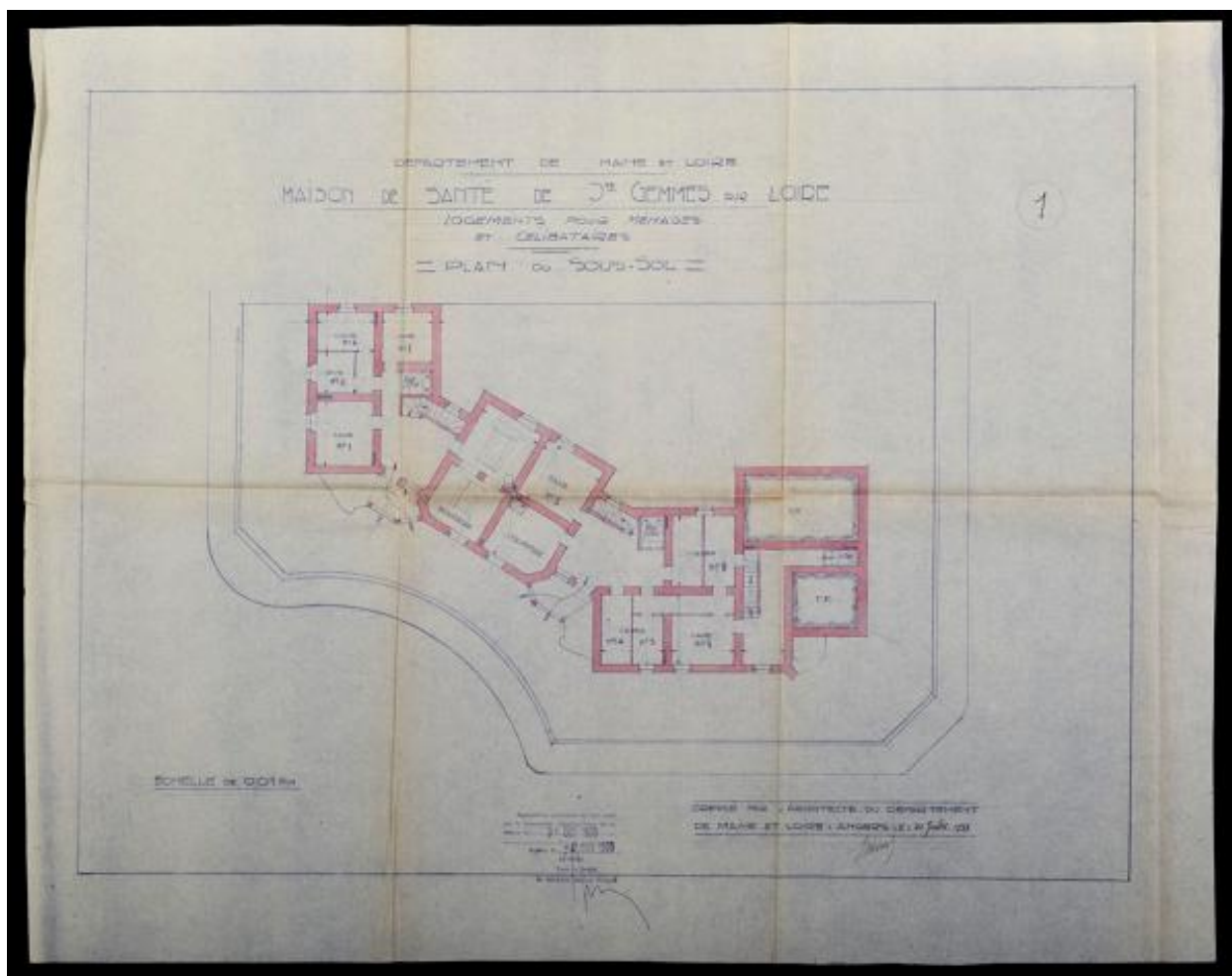
Logements pour célibataires. Plan du sous-sol, par Ernest Bricard. (Archives départementales de Maine-et-Loire, 4 N).
