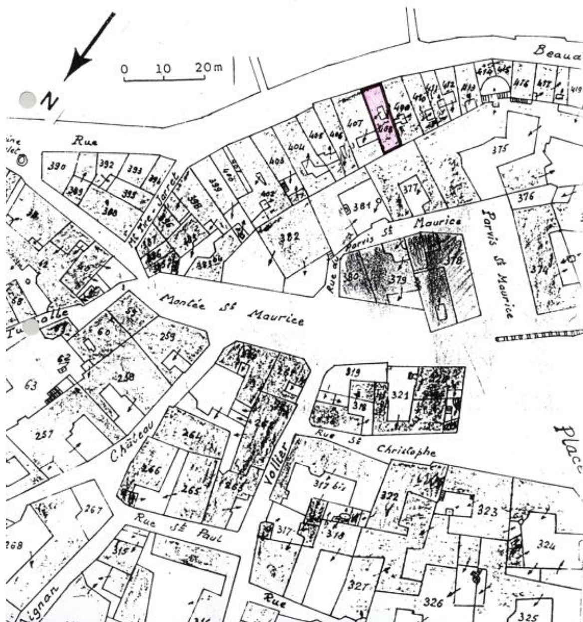
Plan-masse et de situation. D'après le plan cadastral, 1840, section J, parcelle 408, éch. 1 : 1 000, agrandi.
