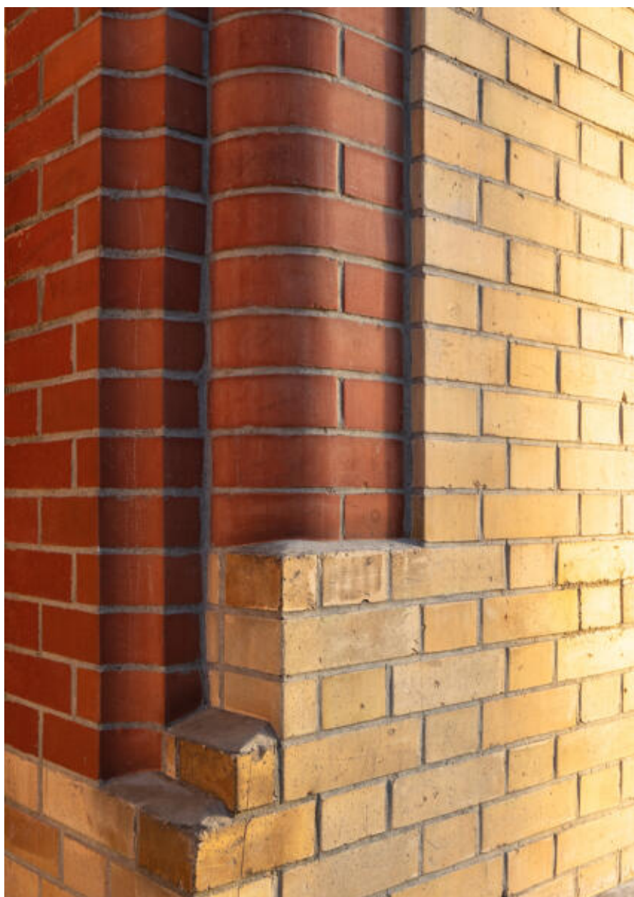
Détail des moulurations du jambage de la porte.
