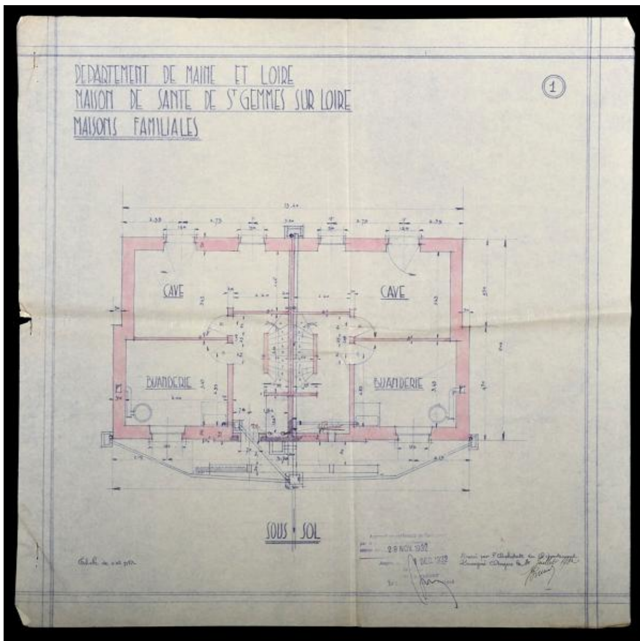
Maisons familiales. Sous-sol, par Ernest Bricard. Juillet 1932. (Archives départementales de Maine-et-Loire, 4 N).
