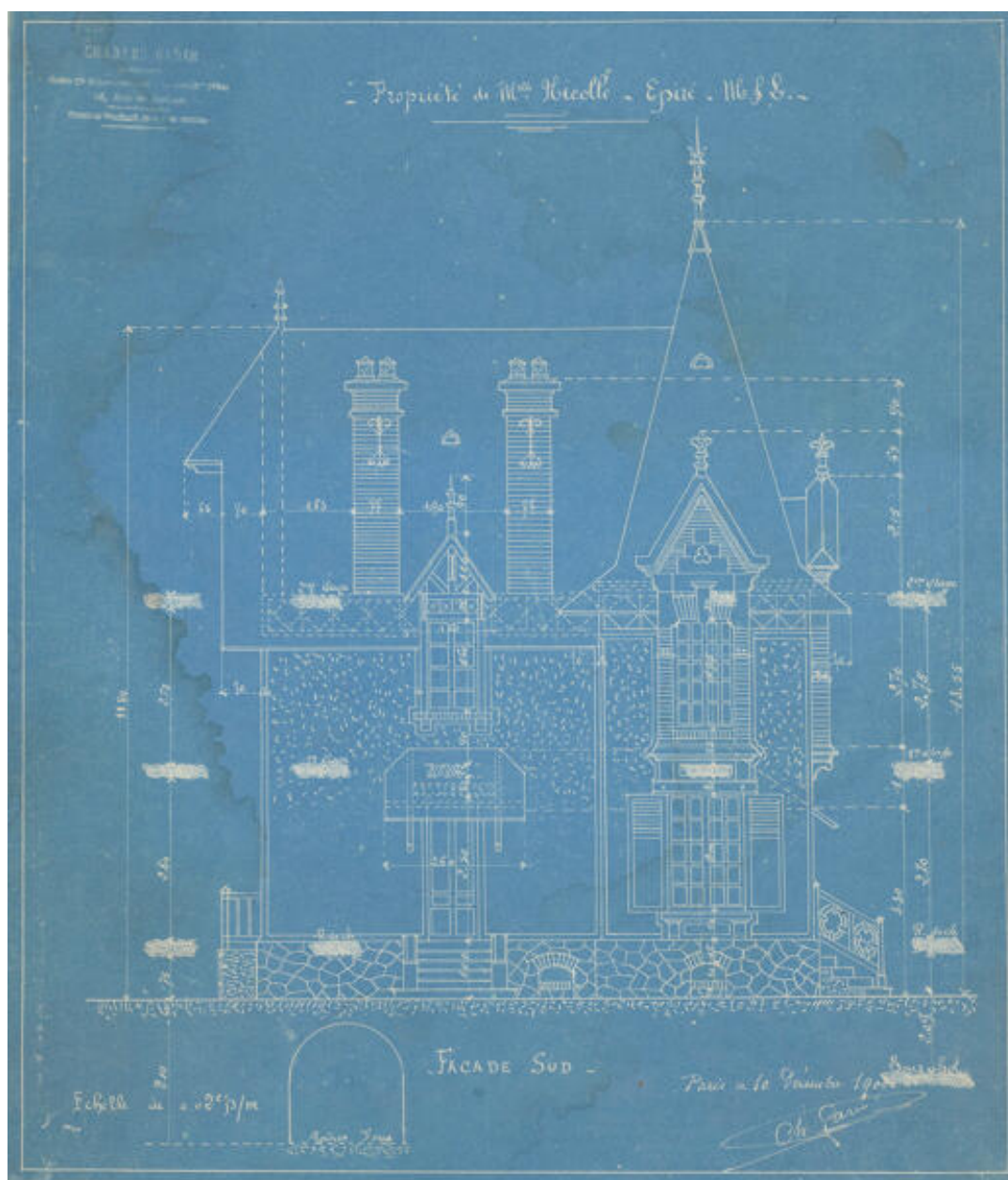
Projet de villa pour Mme Nicolle, par Louis-Charles Garin. Façade sud. Cyanotype, 10 décembre 1900.
