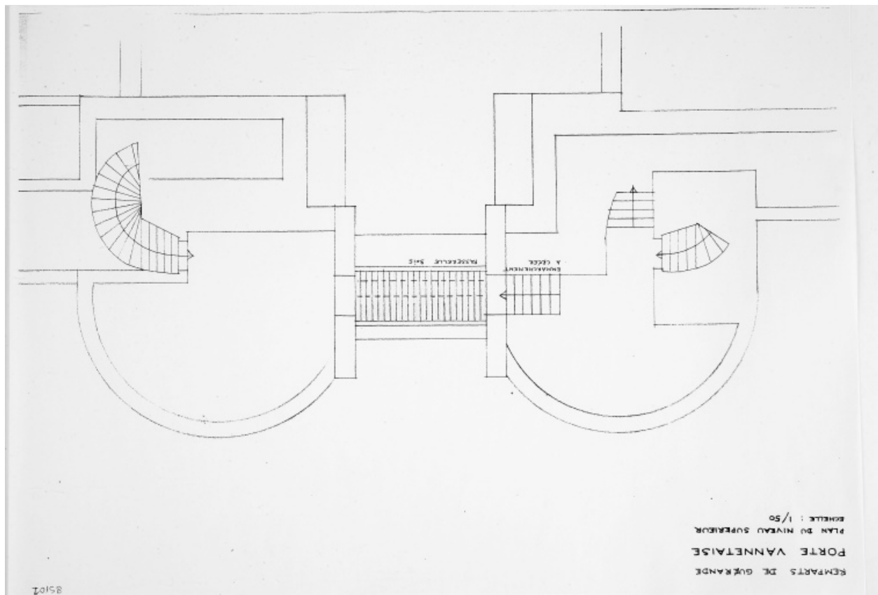
Plan au niveau supérieur.
