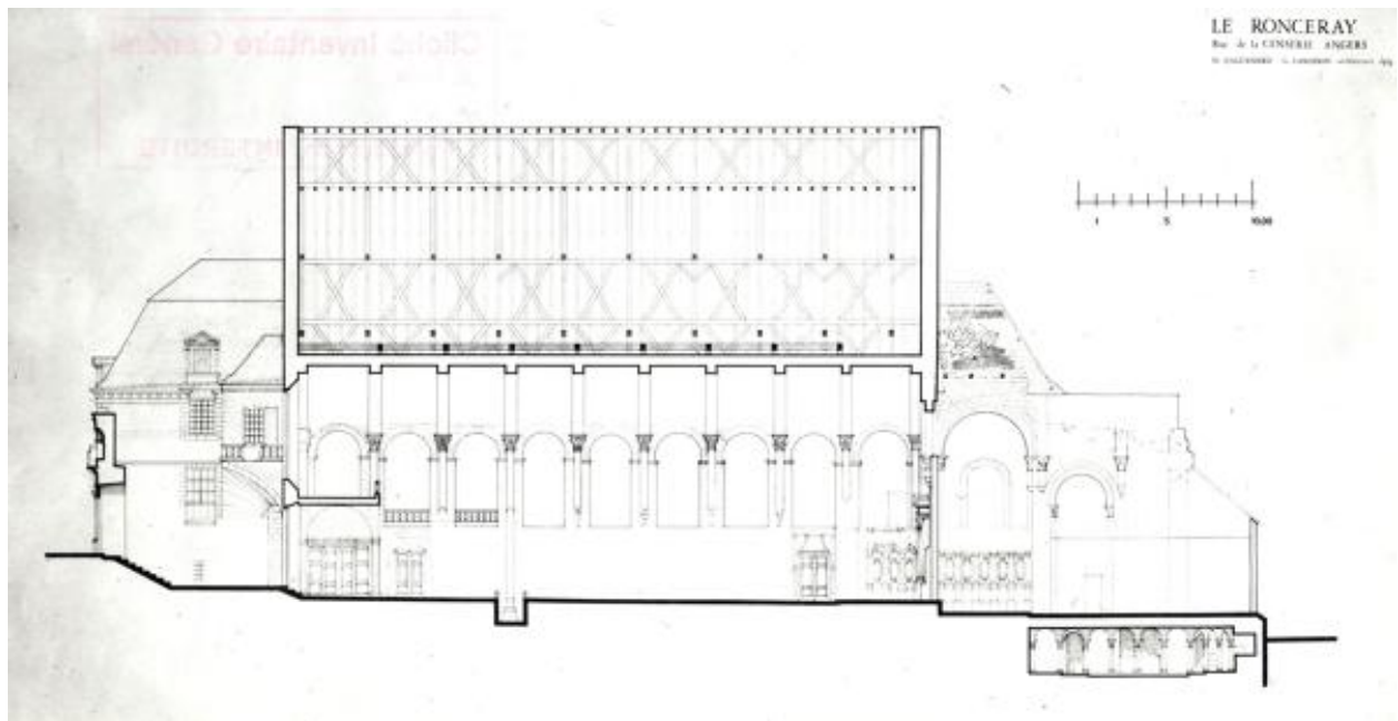
Eglise, coupe longitudinale, par H. Enguehard, [v. 1978].
