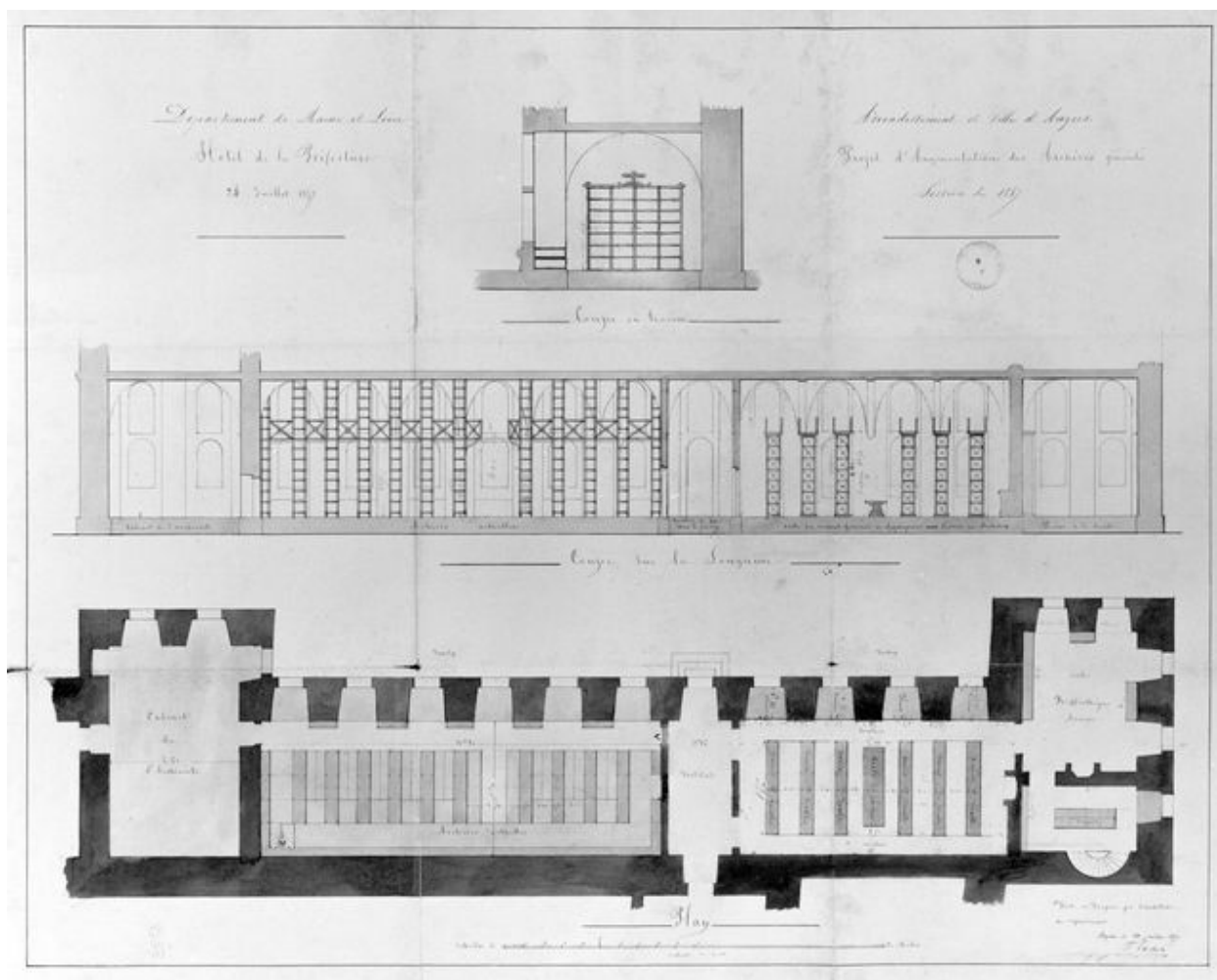
Hôtel de la Préfecture. Projet d'augmentation des Archives générales : coupe en travers, coupe sur la longueur, plan, par l'architecte Ferdinand Lachèse [?], 1857. Relevé aquarellé, 22 juillet 1857, éch. 1 : 100. (Archives départementales de Maine-et-Loire ; N 1773).
