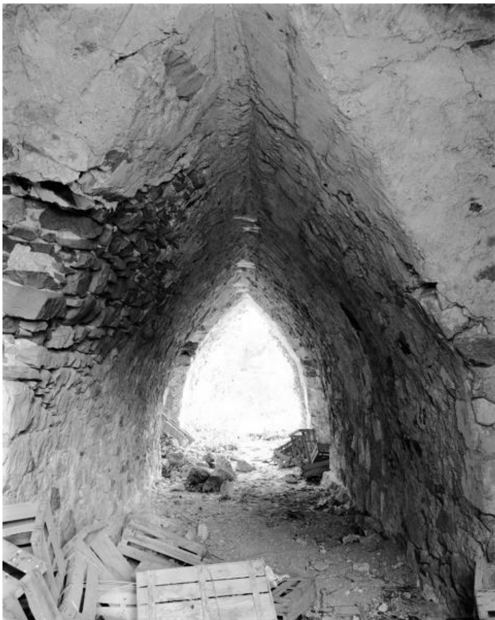
Galerie transversale postérieure (G) du four de Sainte Barbe, vue du nord vers le sud, Montjean-sur-Loire.
