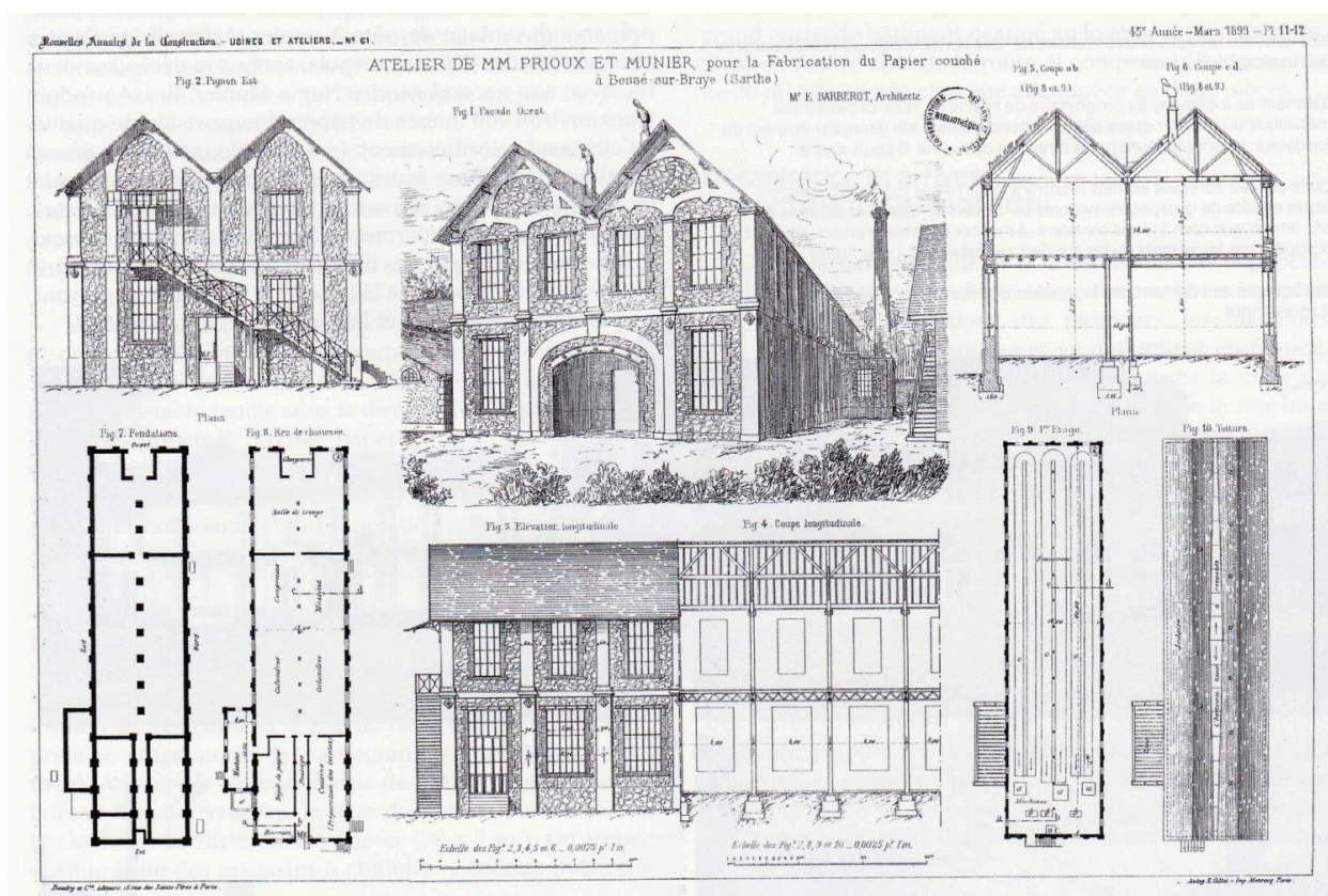
Plans, coupes et élévation de l'atelier de couchage, par Etienne Barberot, architecte. Extrait des Annales de la Construction, 1899. Repro. Louis André / CILAC
