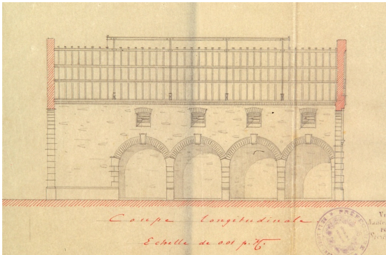
Coupe longitudinale, 1908.
