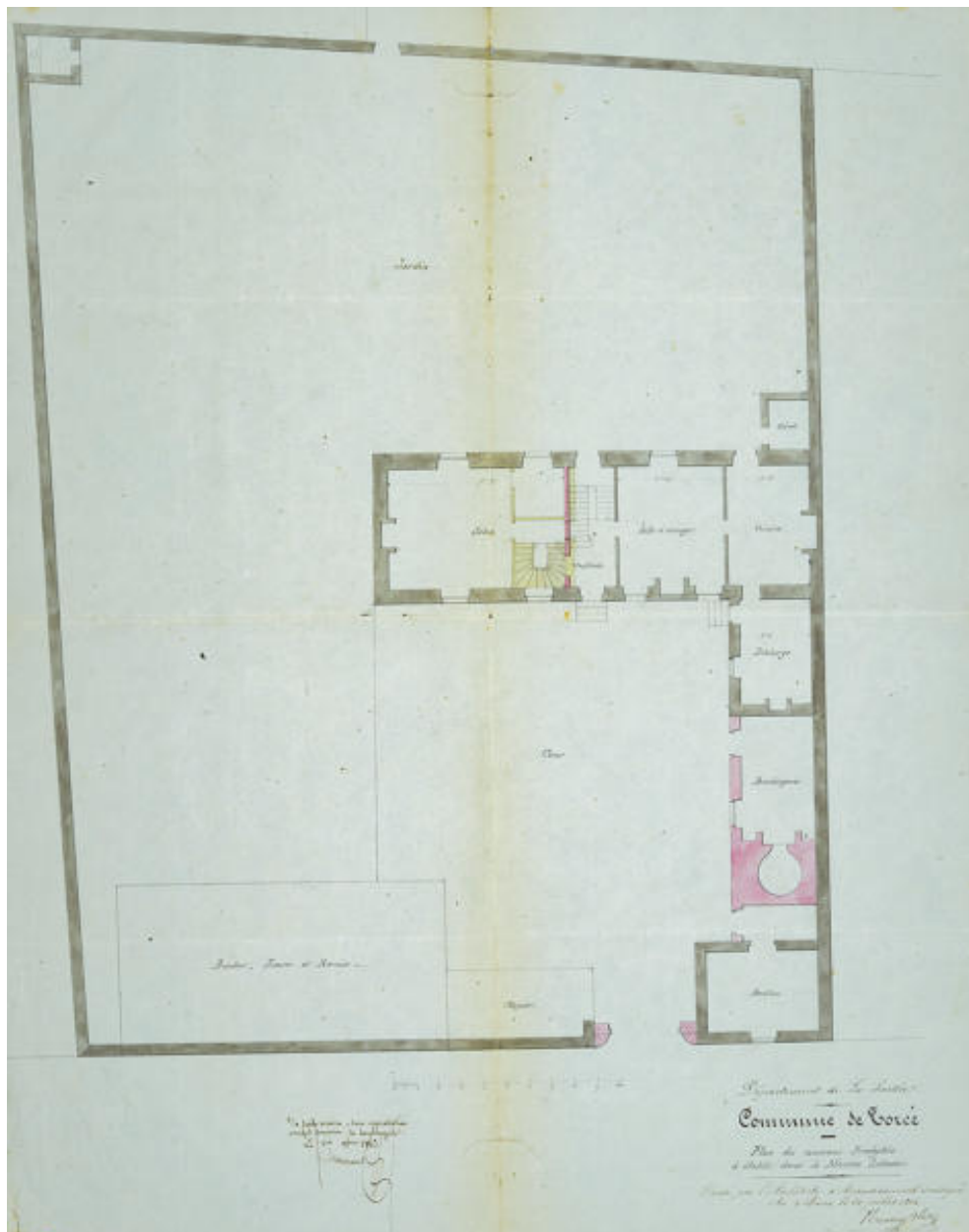
Plan d'aménagement de la maison Letessier en presbytère, 30 juillet 1863.
