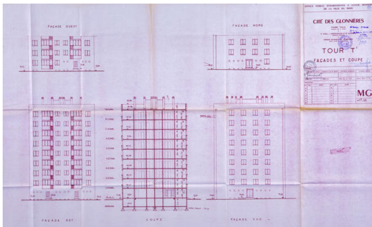
Elévation des façades de la tour 3 des Glonnières.
