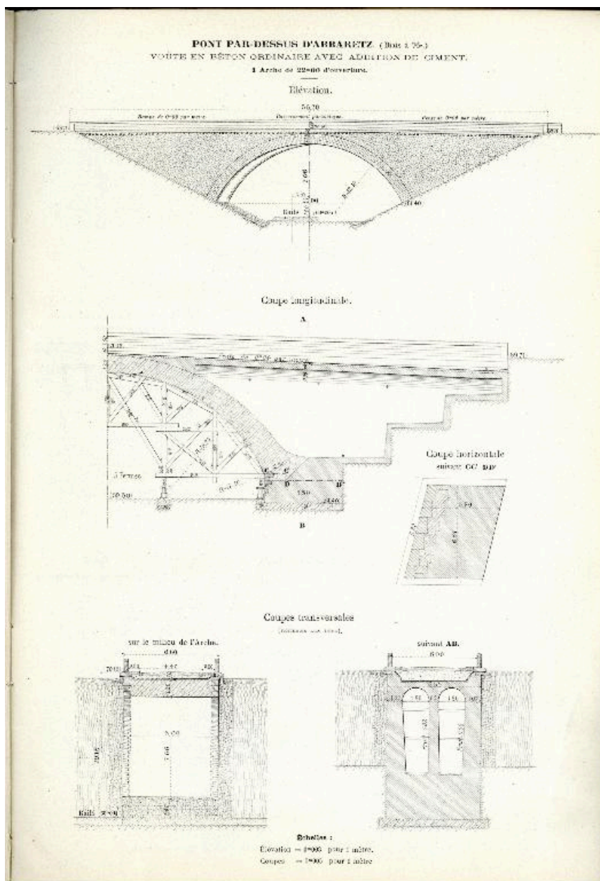
Plan, élévation et coupes de pont-route en voûte de béton de ciment à Abbaretz, 1877.
