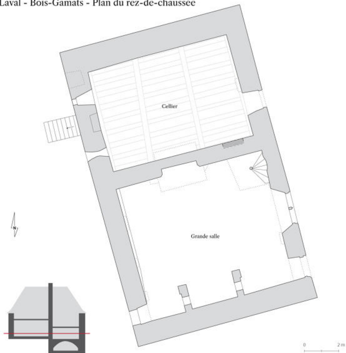
Laval, Bois-Gamats : plan du rez-de-chaussée.
