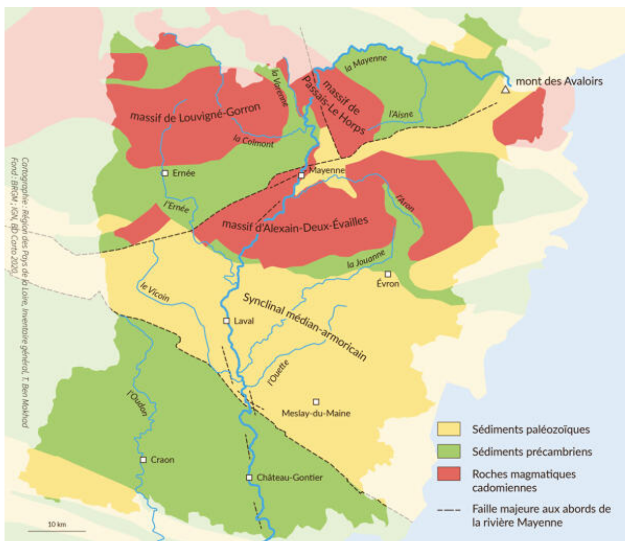
Carte géologique simplifiée du département de la Mayenne.
