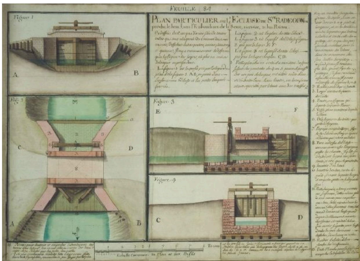
Plan d'une porte ou écluse (ici celle des Grands Greniers) du même type que la porte du canal de l'Epine, par Claude Masse, vers 1700.
