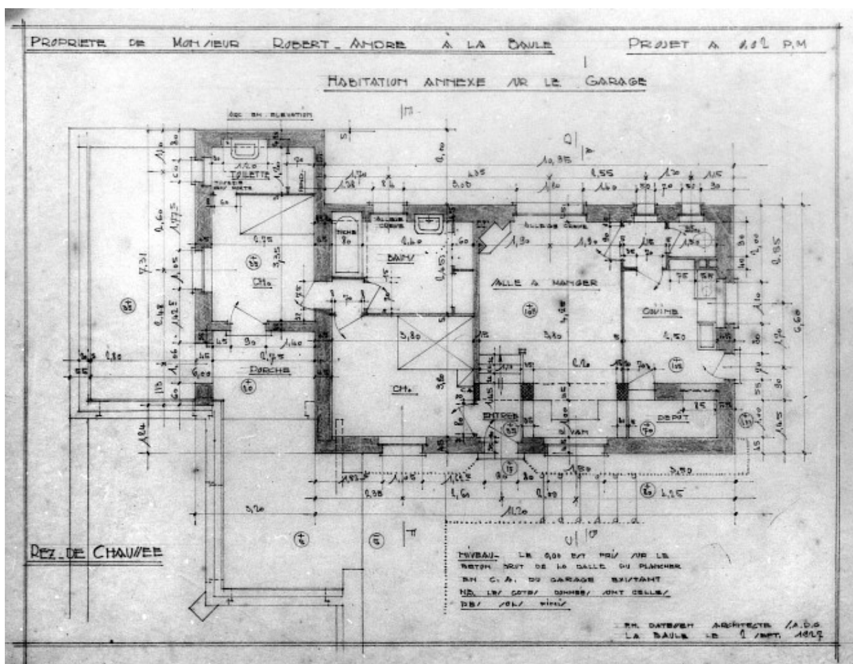
Plan du rez-de-chaussée au 1/50e de la villa Ty Ra Bihan pour M. Robert-André en 1924.
