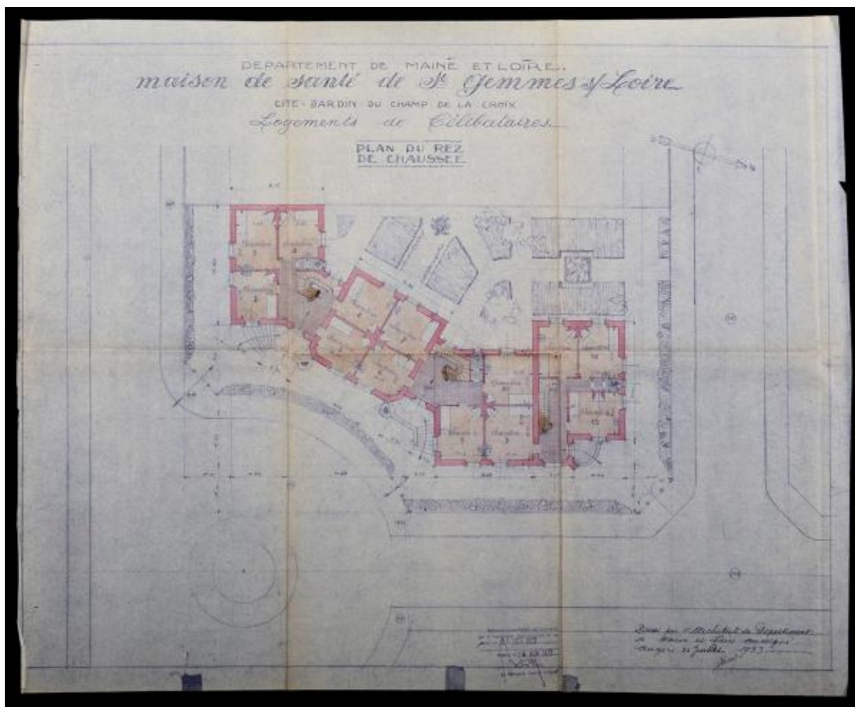
Logements pour célibataires. Plan du rez-de-chaussée, par Ernest Bricard. 30 juillet 1933. (Archives départementales de Maine-et-Loire, 4 N).
