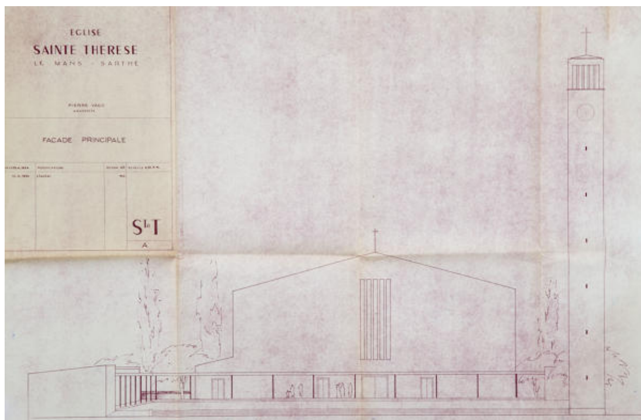
Elévation de la façade principale de l'église Sainte-Thérèse par Pierre Vago.
