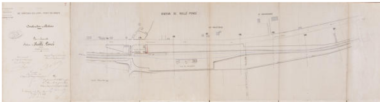
Plan d'ensemble : station de Ruillé-Poncé, 1877.
