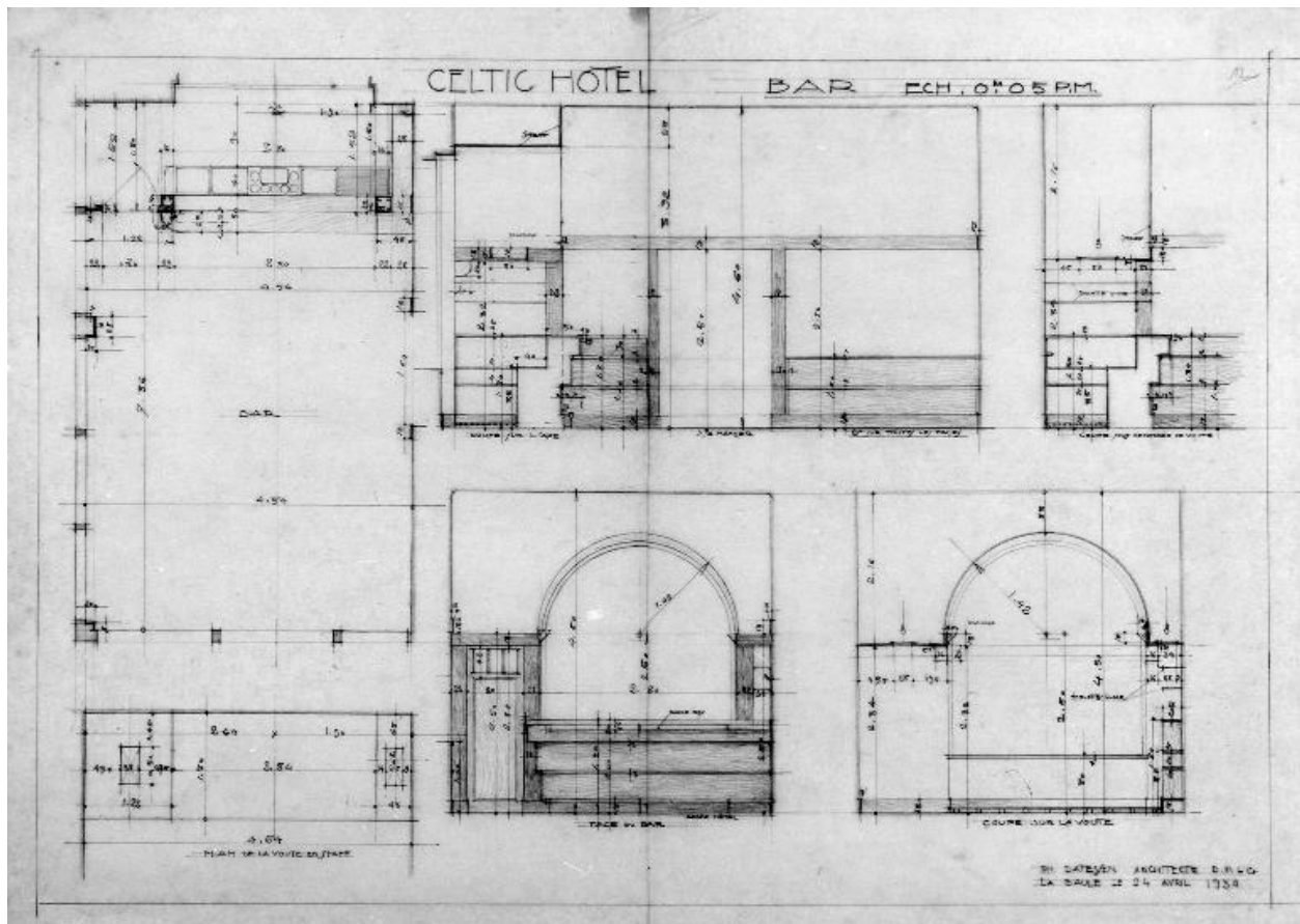
Façades et plan du bar au 1/20e du Celtic Hôtel pour Monsieur Le Gouic en 1930.
