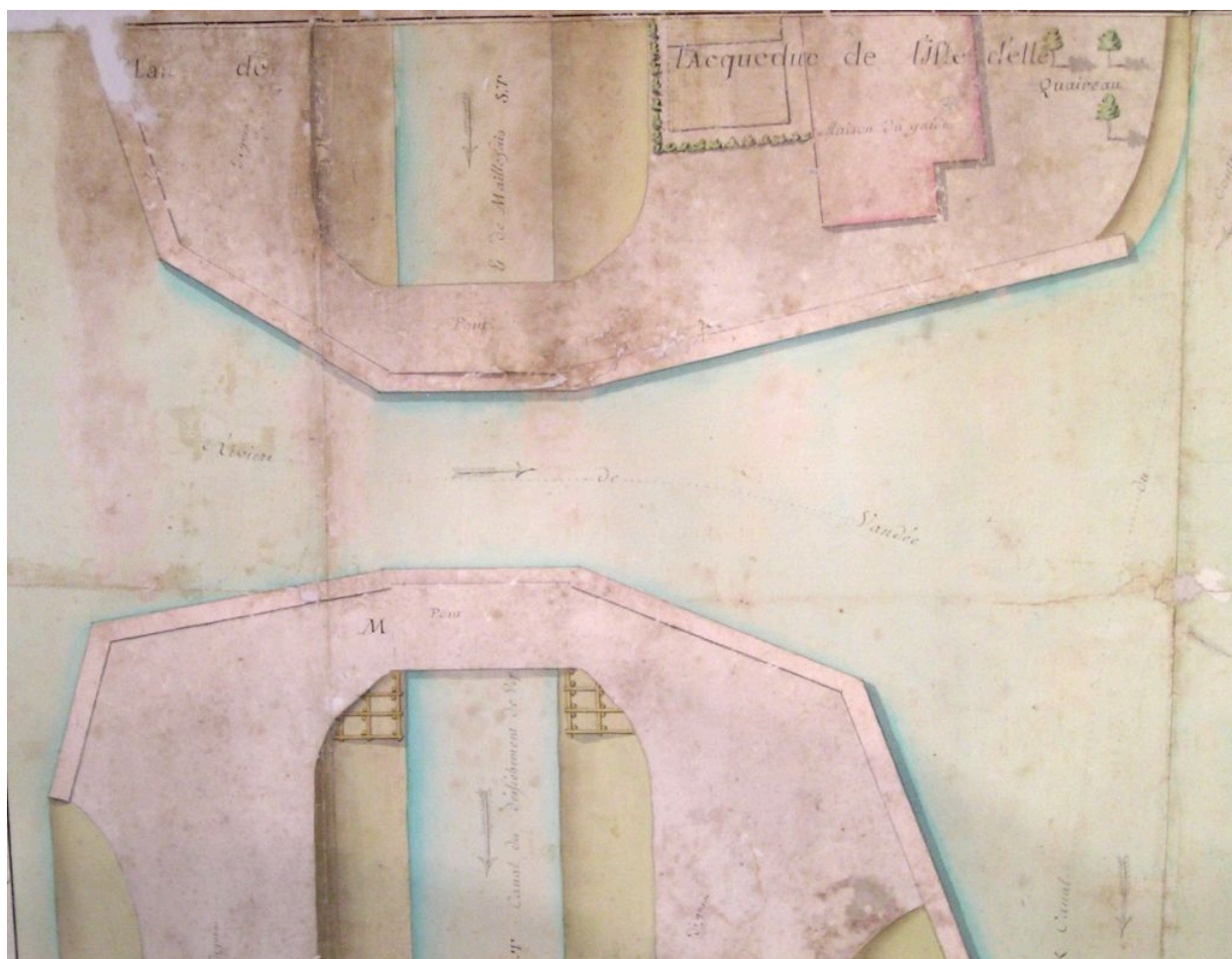
Plan de l'aquaduc du Gouffre par Jacques Parent en 1767.
