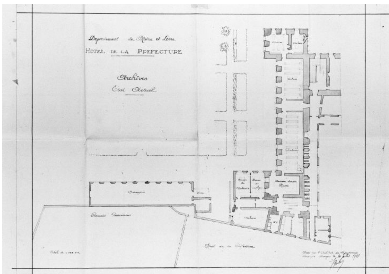
Département de Maine-et-Loire. Hôtel de la Préfecture. Archives. Etat actuel : plan au rez-de-chaussée de l'aile est et de l'orangerie, par l'architecte du département Ernest Bricard, 1933. (Archives départementales de Maine-et-Loire ; N 1773).
