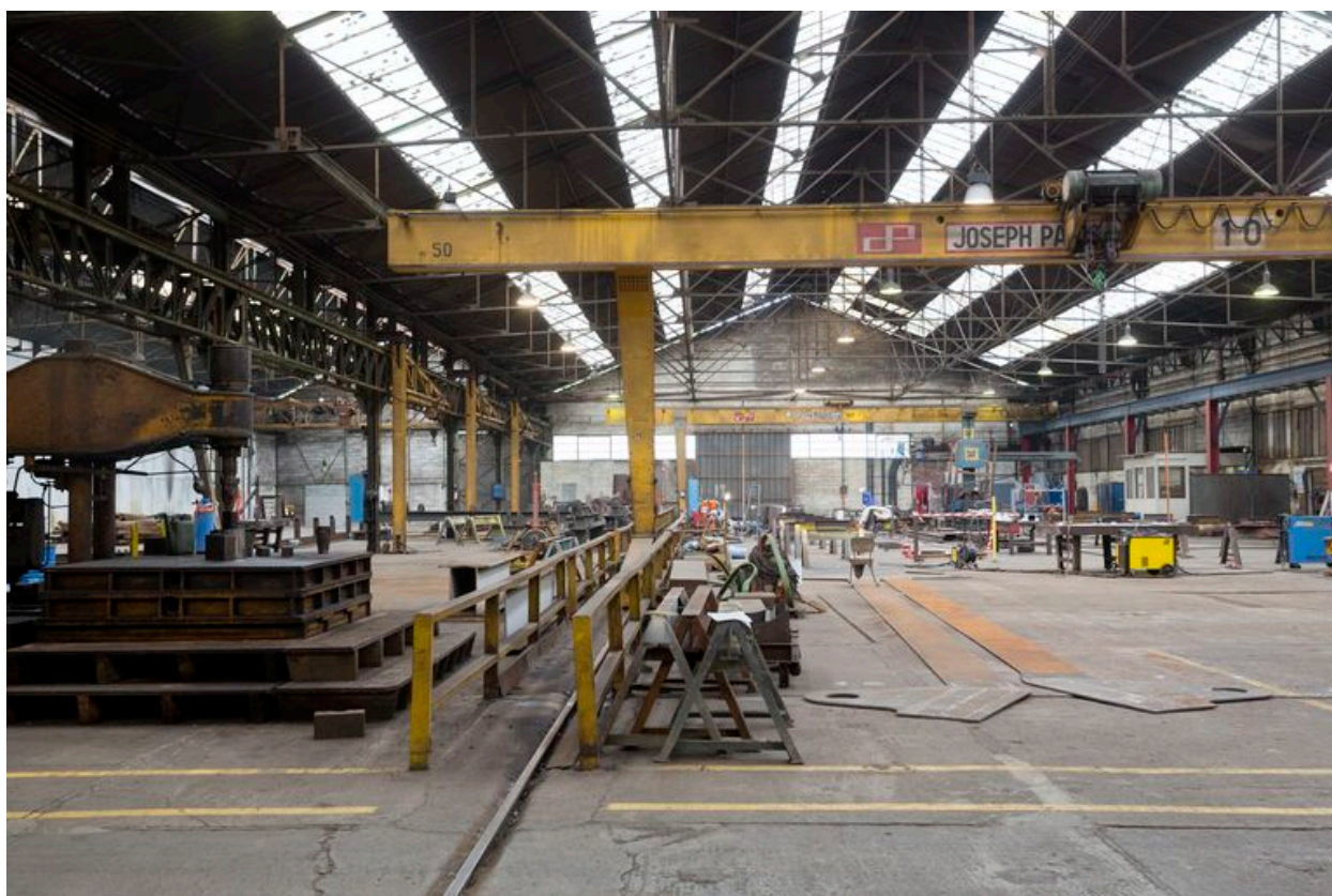
Atelier perpendiculaire à la halle de soudure.
