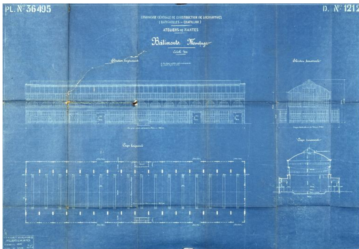
Plan du bâtiment de montage, 1918
