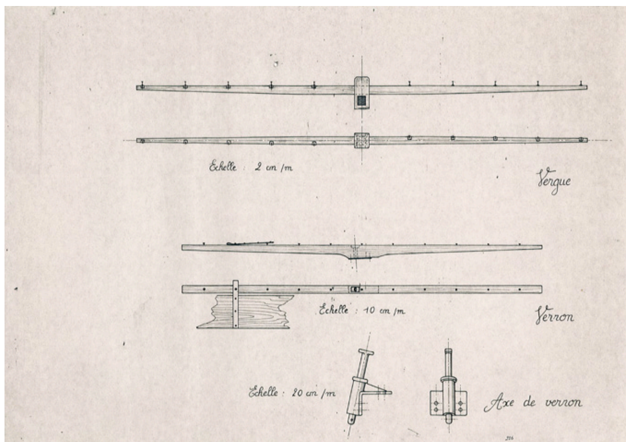
Plan de la vergue et d'un verrou (vers 1980).
