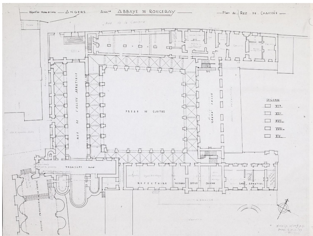
Ancienne abbaye du Ronceray. Plan du rez-de-chaussée, par René Baldet (recenseur MH), tirage de plan, 1977, éch. 1 : 200. 46 x 62 cm.
