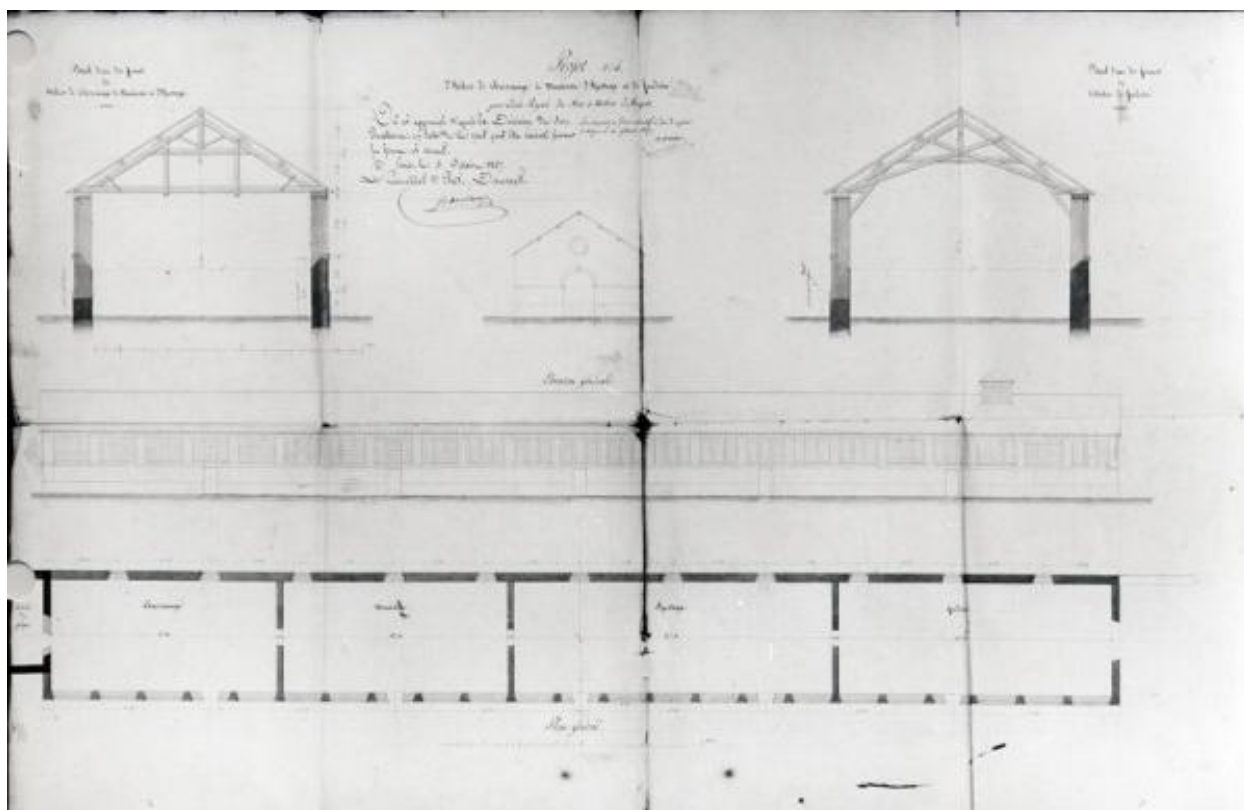
Projet n° 4 d'Ateliers de Charronnage, de Menuiserie, d'Ajustage et de fonderie : plan, coupe transversale, élévations antérieure (sur rue) et latérale, dessin, par B. Bonjour, 1827.
